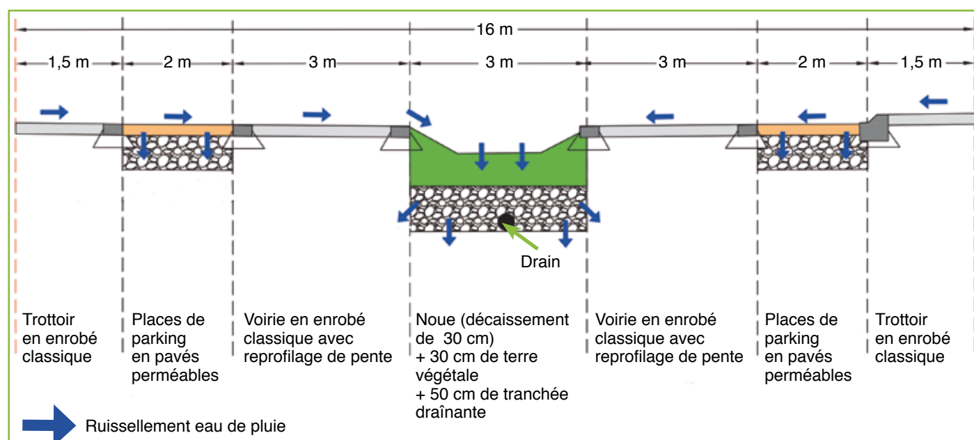
Figure 1 : Coupe de la rue du Donon d'une largeur de 16 m
